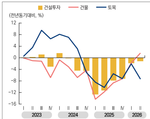
[그림 II-32] 공종별 건설투자 추이
